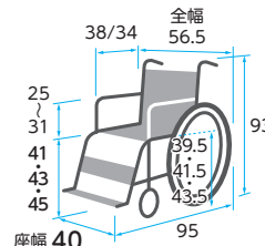
肘掛け高さ調整
